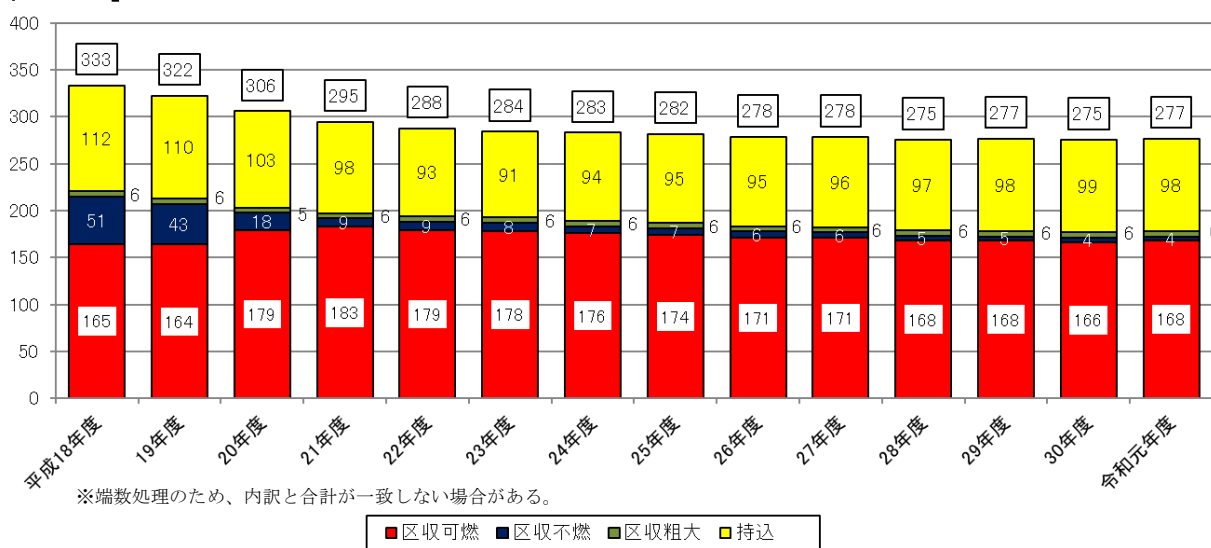
図-1 ごみ量の推移
