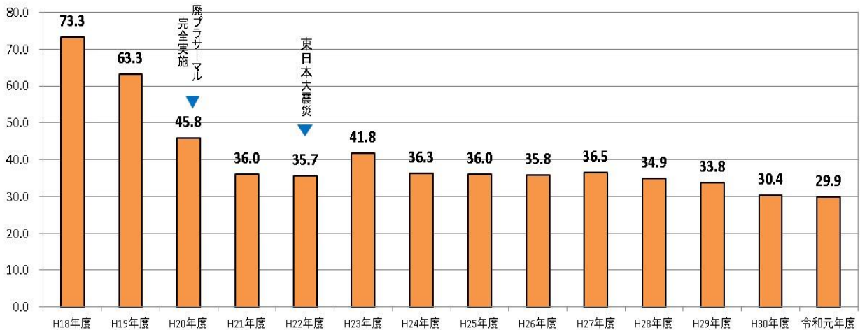
図-5 最終処分量の実績値の推移
