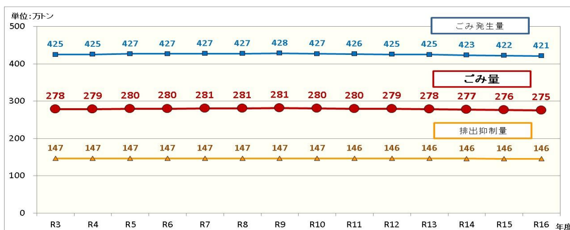
図-2 ごみ量の予測値の推移
